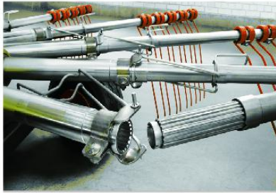
PROFIX 支架使弹齿臂更换便捷, 确保无缝配合, 小磨损连接。
