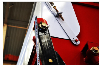
合理设计高度，箱体提至2.3M，更加科学实用，满足多类型车辆，提升运输装卸效能；
